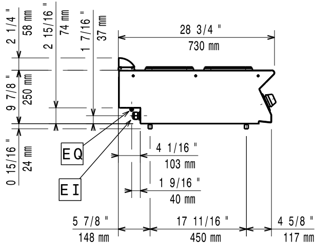
Oldalnézet
