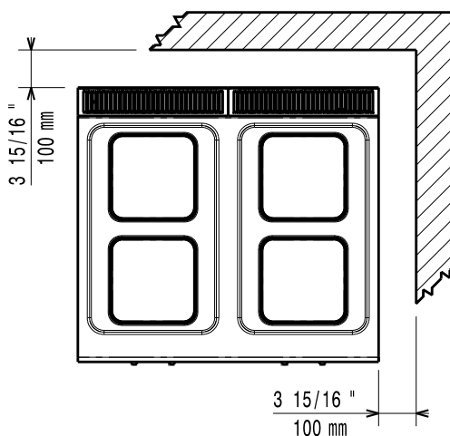
Felülnézet
